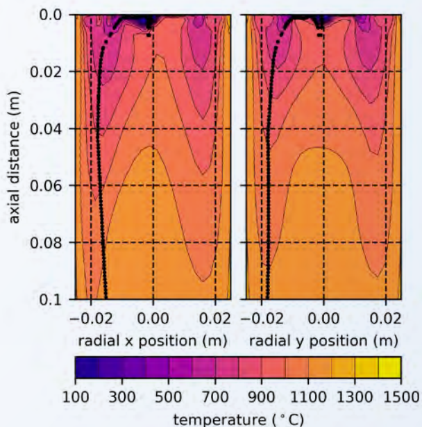
Abb. 16: Temperatur am Kohleinjektionspunkt; die schwarze punktierte Linie zeigt die Partikelbahn (Quelle: TU Wien / K1-MET GmbH).
