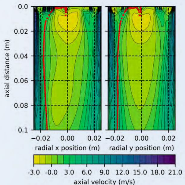
Abb. 17: Geschwindigkeit am Kohleinjektionspunkt; die rote punktierte Linie zeigt die Partikelbahn (Quelle: TU Wien / K1-MET GmbH).
