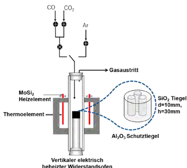
Abb. 2: Schematische Darstellung des Widerstandsofens für die experimentellen Versuche (Quelle: K1-MET GmbH).
