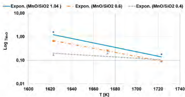
Abb. 5: Berechnete Aktivitätskoeffizienten (Quelle: K1-MET GmbH).
