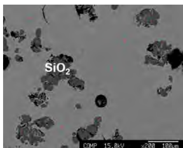
Abb. 4: Schlackenanalyse nach dem Equilibriums-Versuch bei 1350 °C (Quelle: Universität Tohoku).
