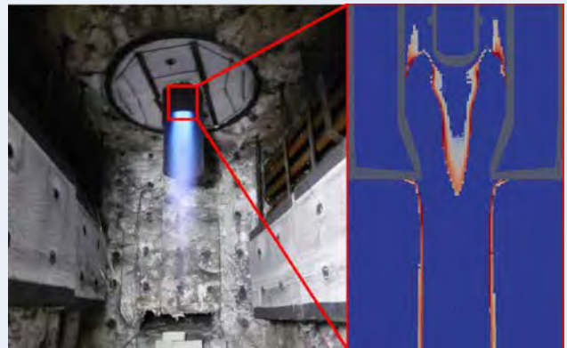
Abb. 15: Bildungszonen von Stickstoffmonoxid in einem industriellen Brenner (Quelle: Montanuniversität Leoben / K1-MET GmbH).
