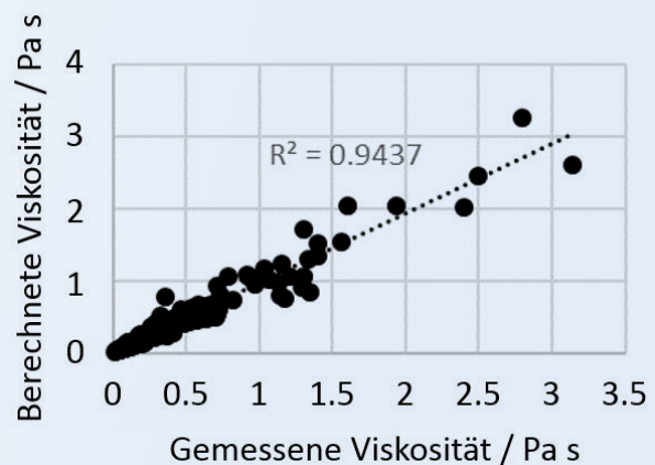
Abb. 14: Vergleich berechneter Schlackenviskositätswerte (Verwendung von KNN) mit gemessenen Daten (Quelle: Montanuniversität Leoben / K1-MET GmbH).
