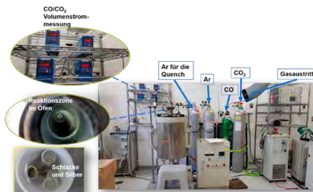
Abb. 3: Experimenteller Versuchsaufbau (Quelle: Universität Tohoku).
